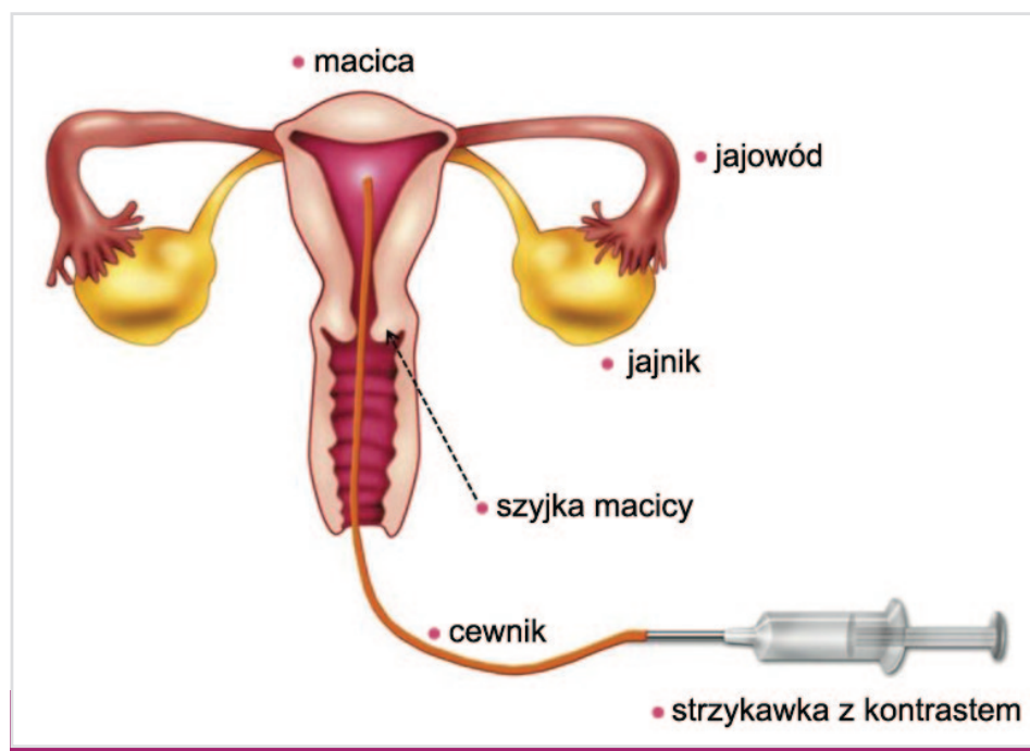
Rys.1 - Zabieg HyCoSy
